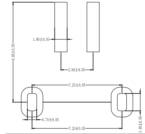
参考PCB板
